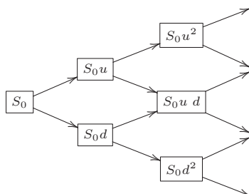
Rys. 1. Drzewo dwumianowe
