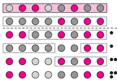
Rys. 5. Przykładowy zestaw kolorów zerowych dla kodu (nad linią) oraz praktyczna realizacja czterech pytań z rysunku 4 z wykorzystaniem tego zestawu (pod linią). Zauważmy, że trafność pytań pozostała niezmienną. Szare ramki obejmują szpilki będące teoretycznie koloru zerowego.
