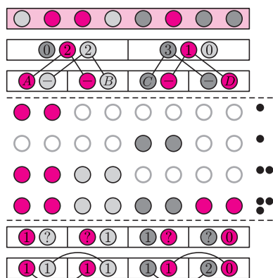
Rys. 4. Przebieg jednej gry w monety podczas trzeciego kroku algorytmu. Wagi monet dla bloków B_1, B_2 są już znane; chcemy ustalić wagi ich pod-monet, których jest 8. Wybieramy 4 z nich (po jednej w każdym bloku) i znajdujemy ich wagi A, B, C, D , zadając pytania odpowiadające ważeniom
