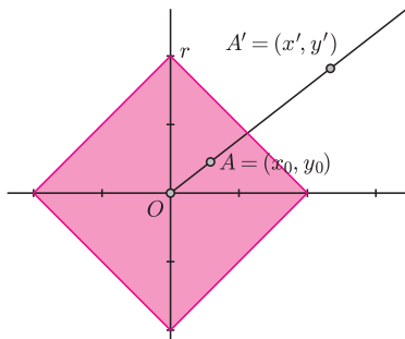
Rys. 1. Okrąg w metryce miejskiej
