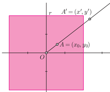
Rys. 2. Okrąg w metryce maximum
