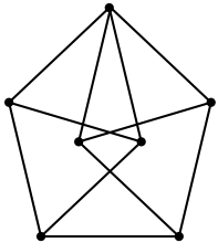
Rys. 2. Wrzeczono Mosera: 7 wierzchołków, wszystkie krawędzie długości 1.
