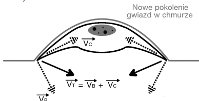
Rys. 2. Zmiana kształtu chmury pyłowej pod wpływem uderzenia fali promieniowania UV. Krańce chmury zaczynają się uginać z powodu powstania zagęszczonego obszaru w centrum chmury, gdzie zaczynają tworzyć się nowe gwiazdy
